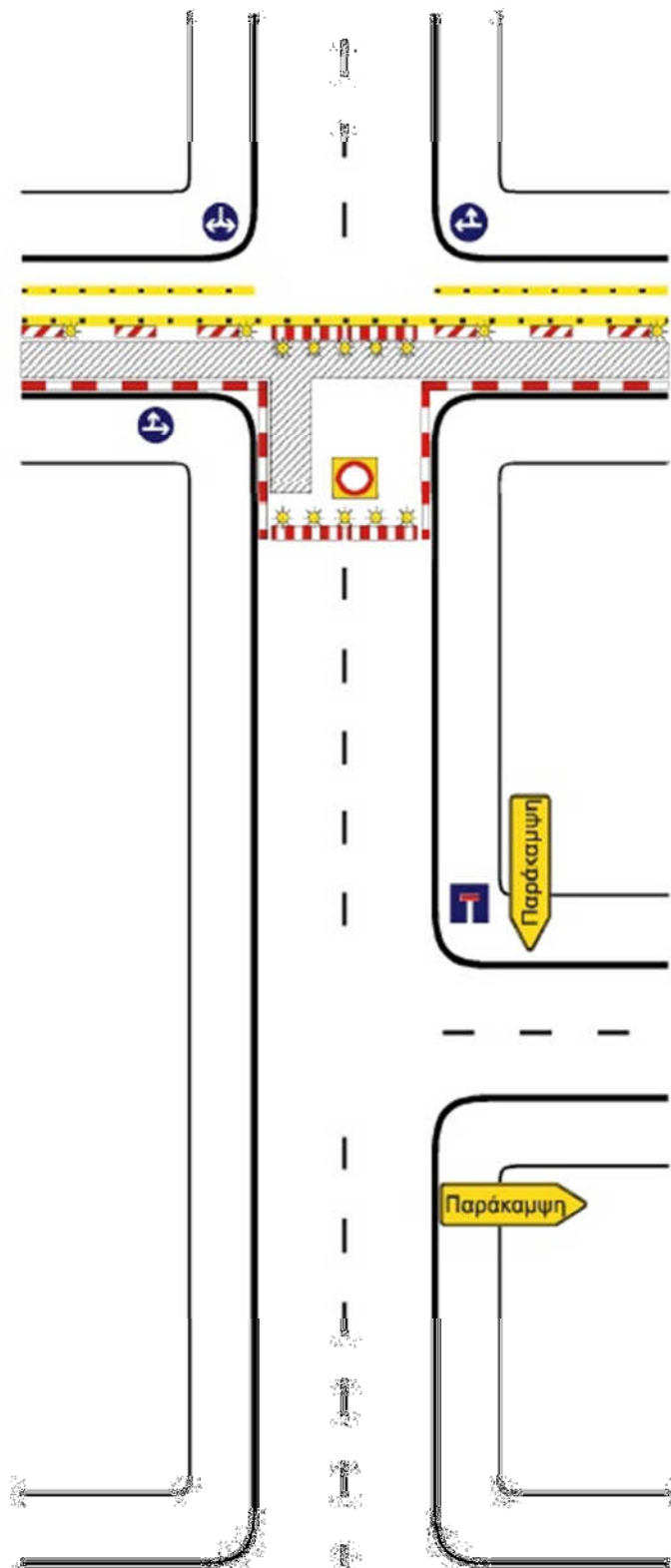
Σχήμα 3.1.4: Εργασίες σε περιοχή συμβολής οδών με αποκλεισμό πρόσβασης.
