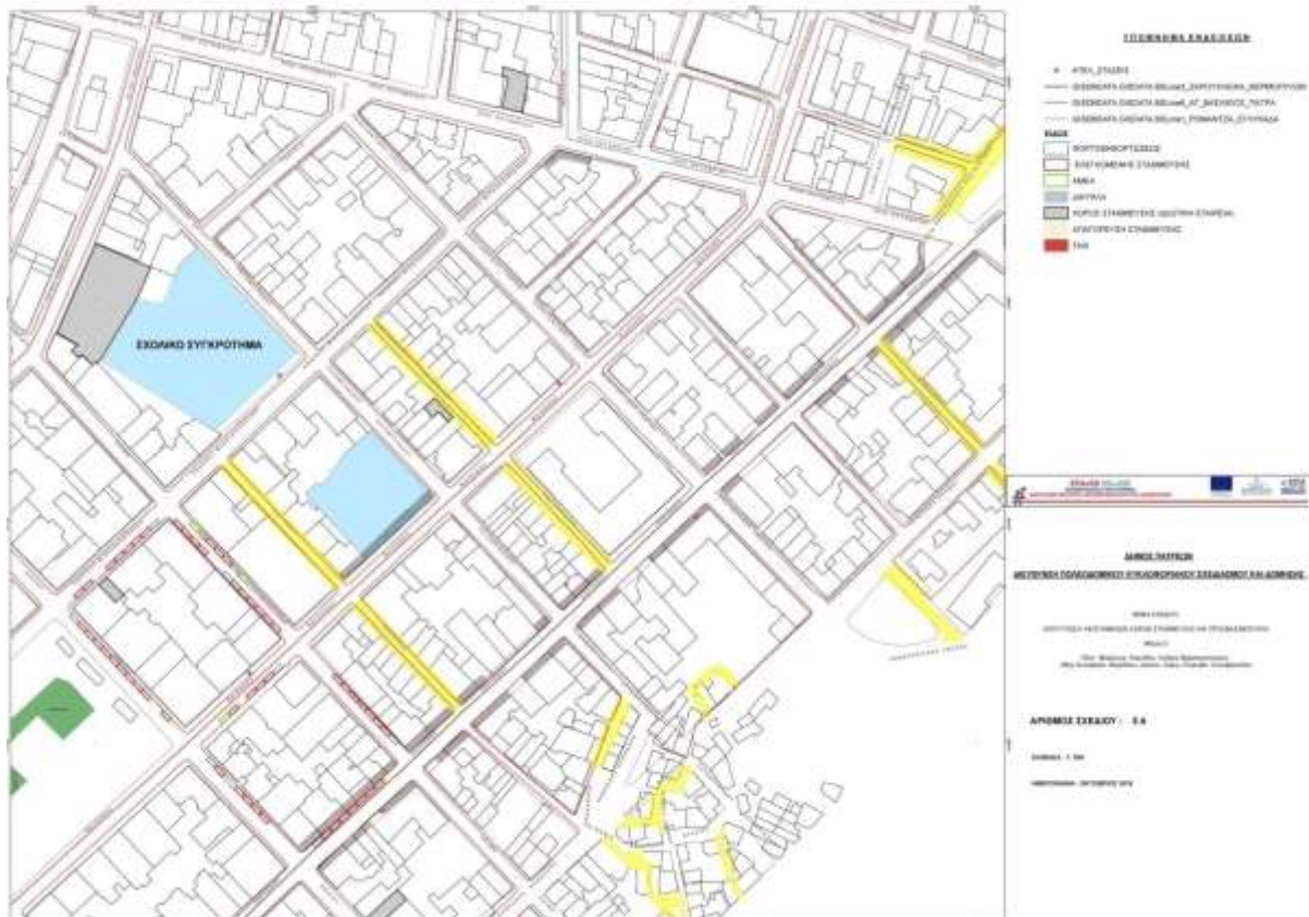
Χάρτης 5: Θέσεις ασύρματου αισθητήρα ελέγχου θέσης στάθμευσης
